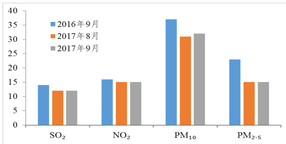
图 1 云南省环境空气主要污染物月均值变化情况 (单位: \mu\text{g}/\text{m}^3 )
